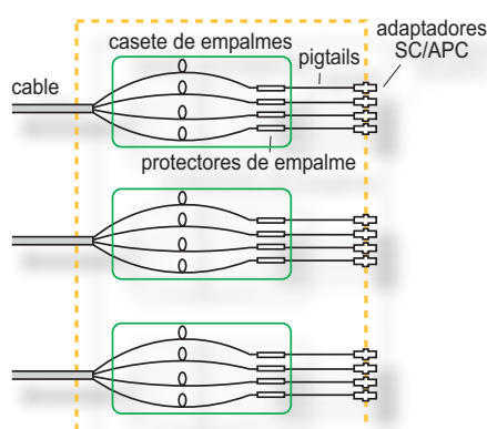
Diagrama de montaje de FKH-312.
